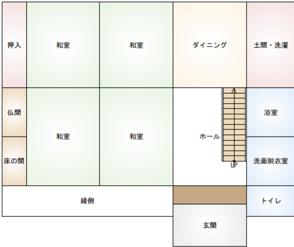
1階間取り図
