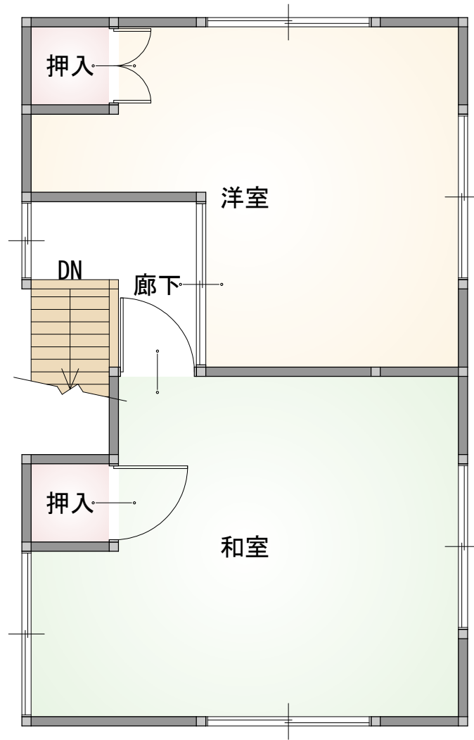
2階平面図
