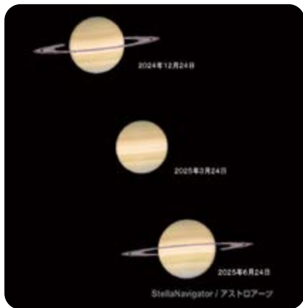
▲リングが見えなくなる土星のようす (株式会社アストロアーツホームページから転載)
