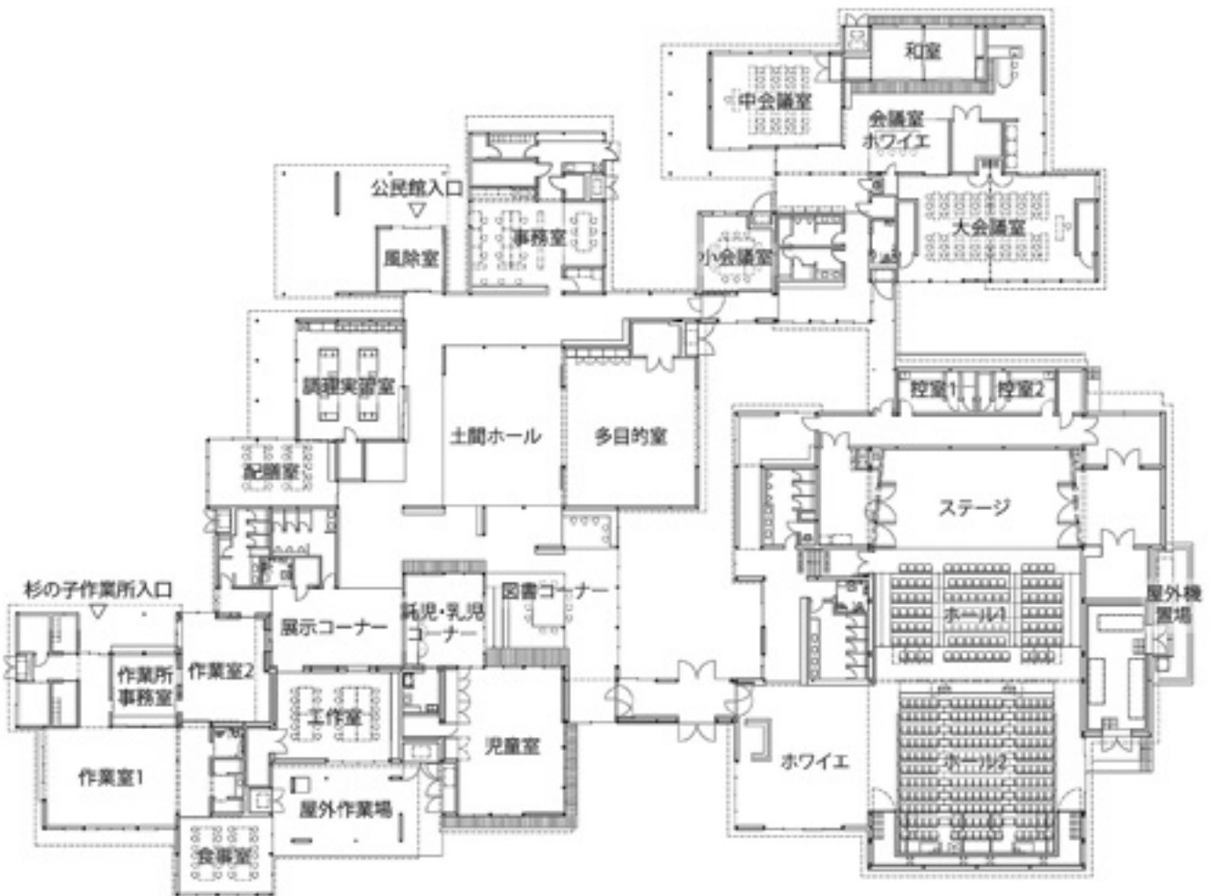
▲新中央公民館の平面図
